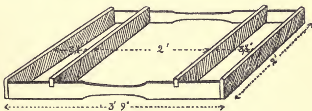
Fig. 7. Cloche-Carrier.
